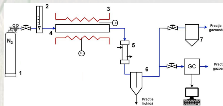
Piroliză
